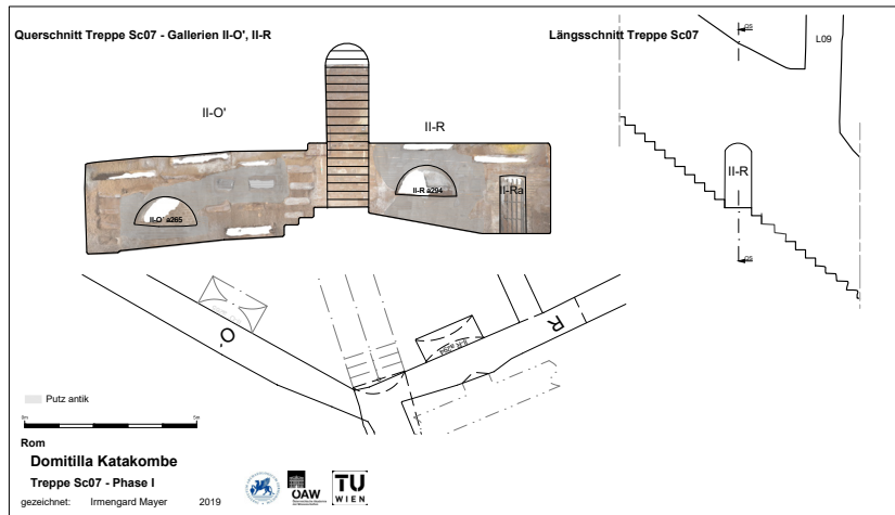
19 Domitilla-Katakombe. Treppe Sc07, Rekonstruktion Phase I, Wandansicht und Plan. (Grafik: N. Zimmermann, I. Mayer/ÖAW)
