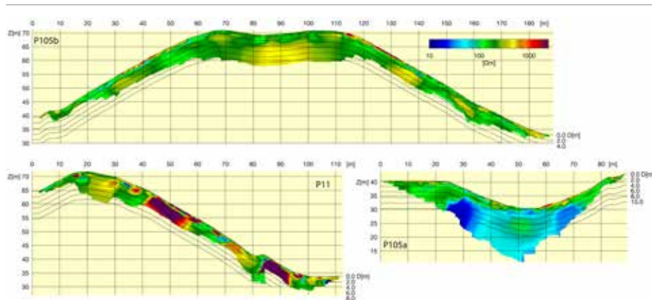
13 Pergamon, Yiğma Tepe. Beispiele geoelektrischer Transekte. Farblich dargestellt ist die durch elektrische Widerstandstomographie ermittelte räumliche Verteilung des spezifischen elektrischen Bodenwiderstands (Abb.: R. Mecking – E. Erkul – W. Rabbel).
