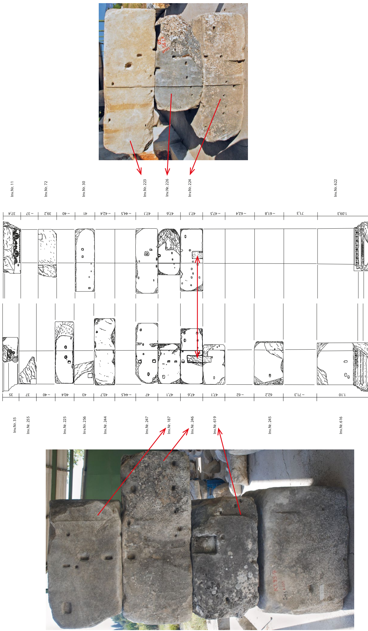
Abb. 13: Lagina, Hekate-Tempel. Innenseite der beiden Anten mit Stifflöchern und Einarbeitungen für einen nachträglich eingefügten Türsturz (M. 1 : 50)
