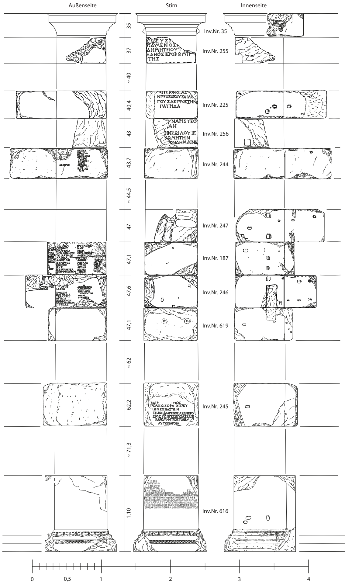
Abb. 1: Lagina, Hekate-Tempel. Rekonstruktion der linken Ante (M. 1 : 33⅓)
