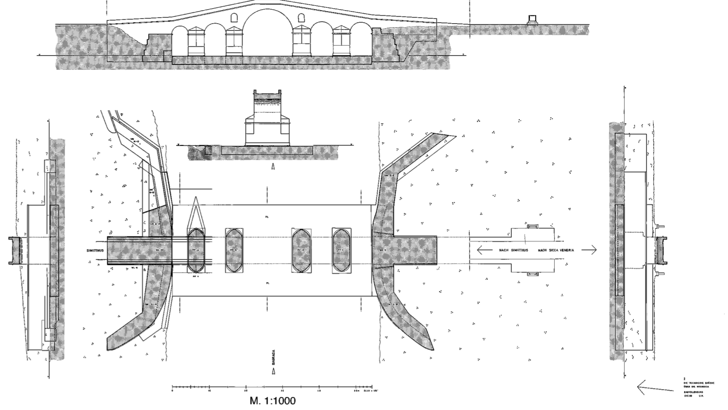
Rekonstruktionsvorschlag: pons novus (2. Phase)
