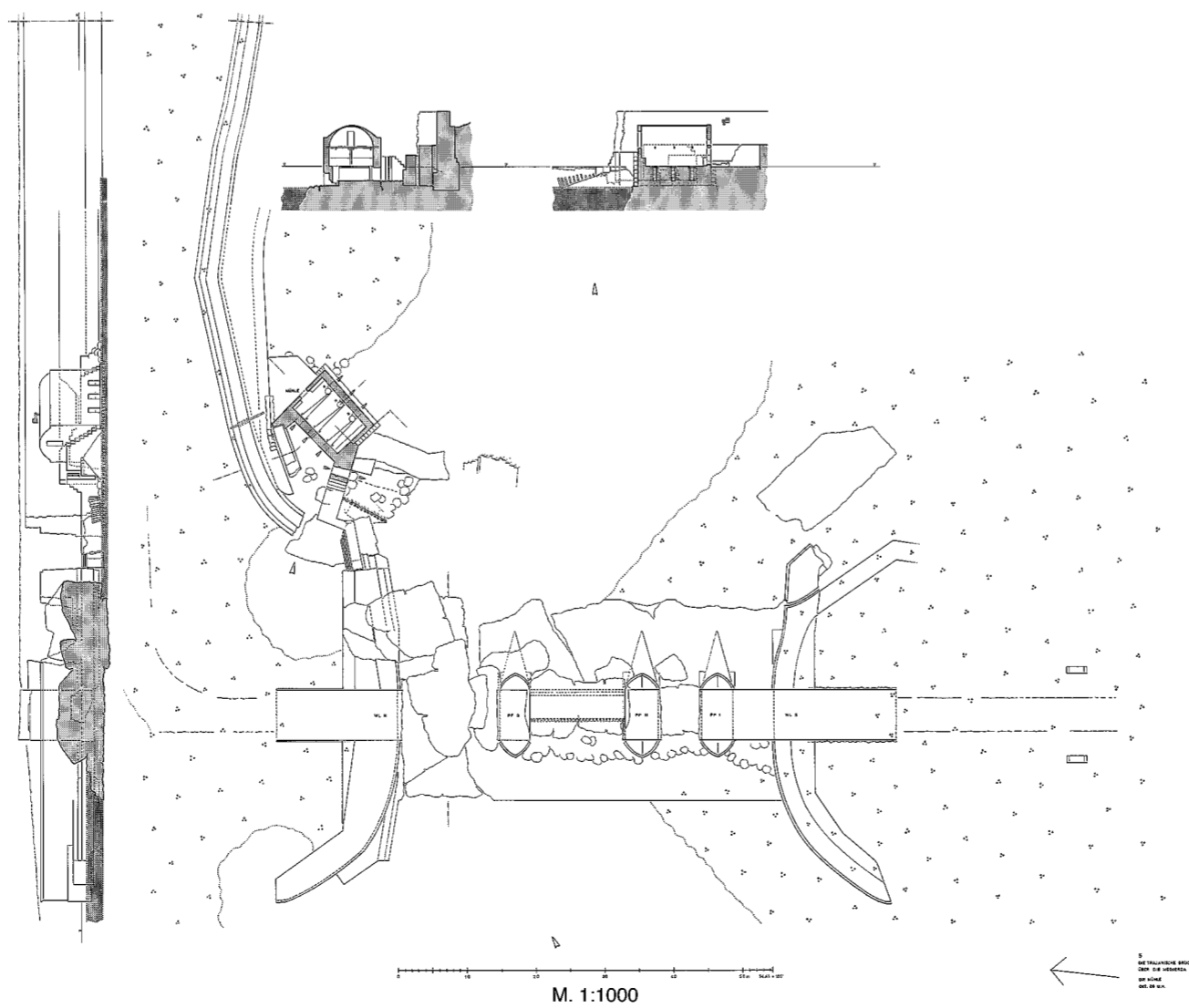
Rekonstruktionsvorschlag: die Brücke nach ihrer Zerstörung (5. Phase)
