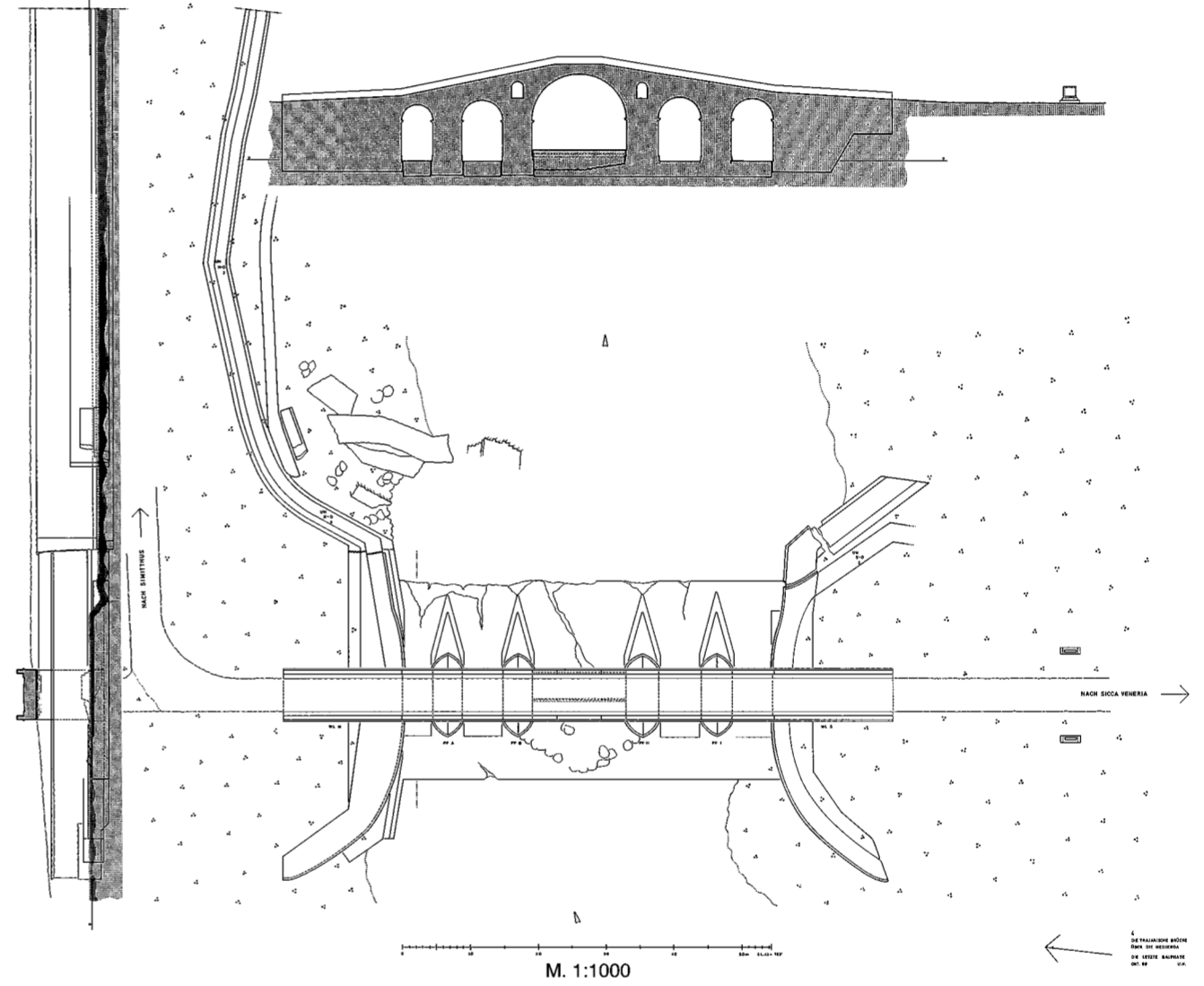
Rekonstruktionsvorschlag: »große Reparaturphase« (4. Phase)
