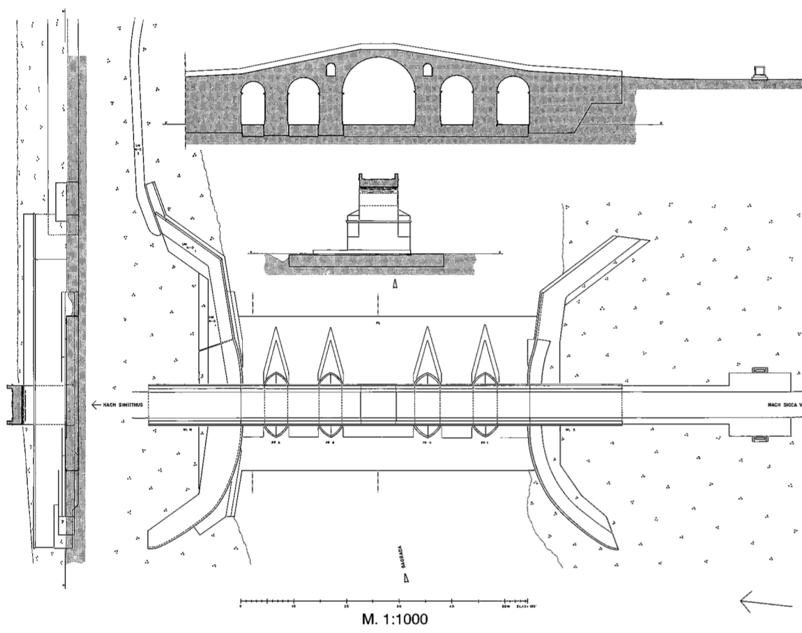
Rekonstruktionsvorschlag: »erste Reparaturphase« (3. Phase)
