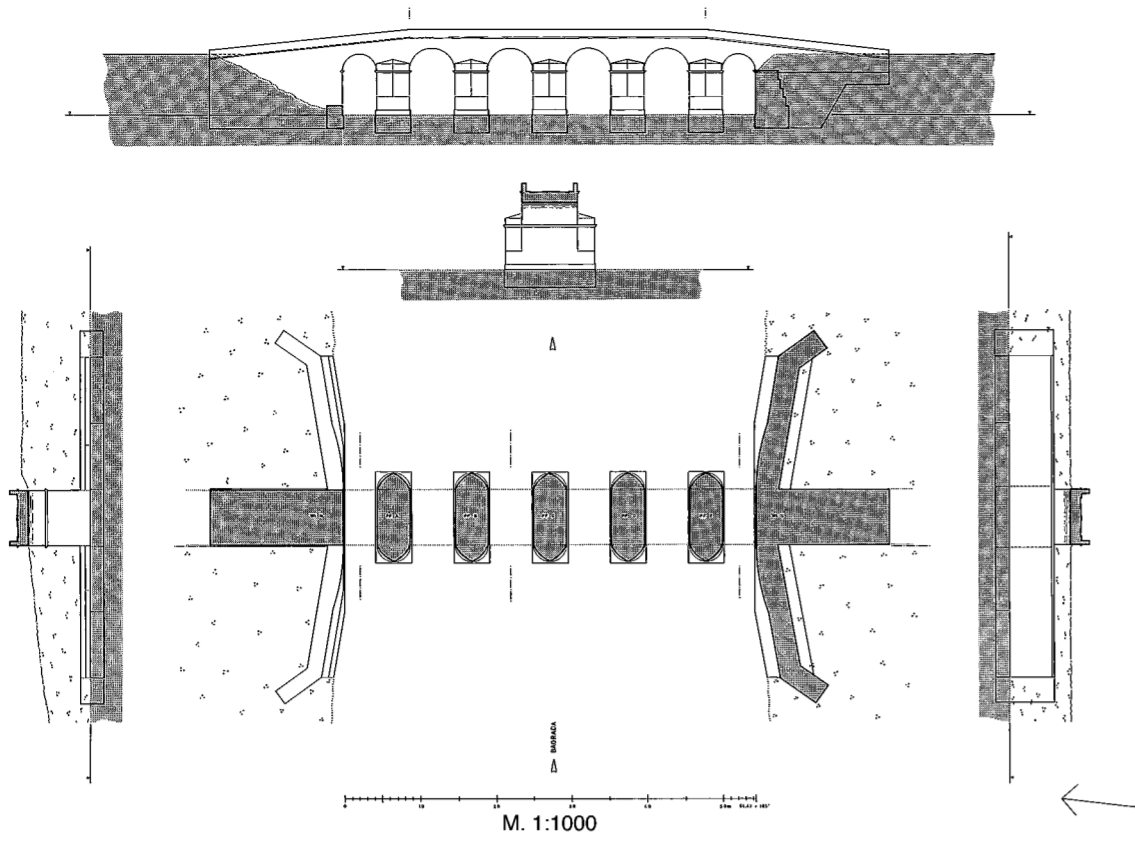
Rekonstruktionsvorschlag: »erste Brückenplanung« (1. Phase)
