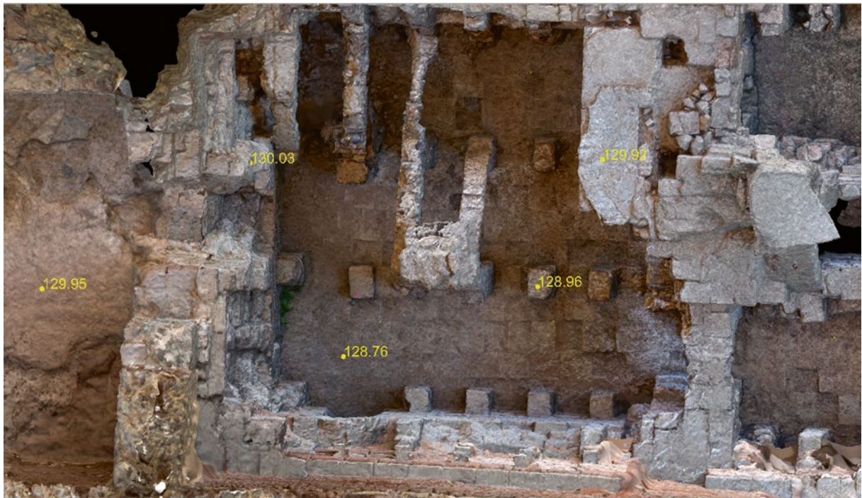
2 Absolute Höhenangaben im 3D-Modell.
