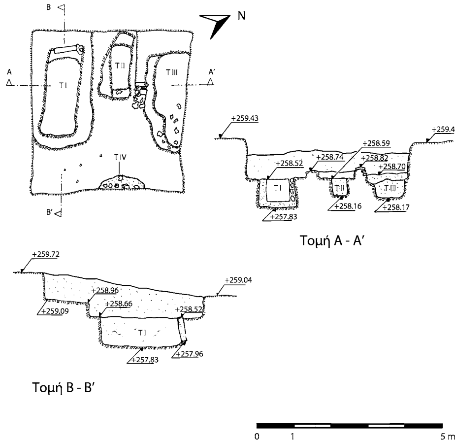
3 Τάφοι I-IV. Κάτοψη και τομές (κλ. 1:100)
