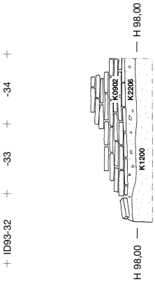
Abb. 57: Nordprofil
